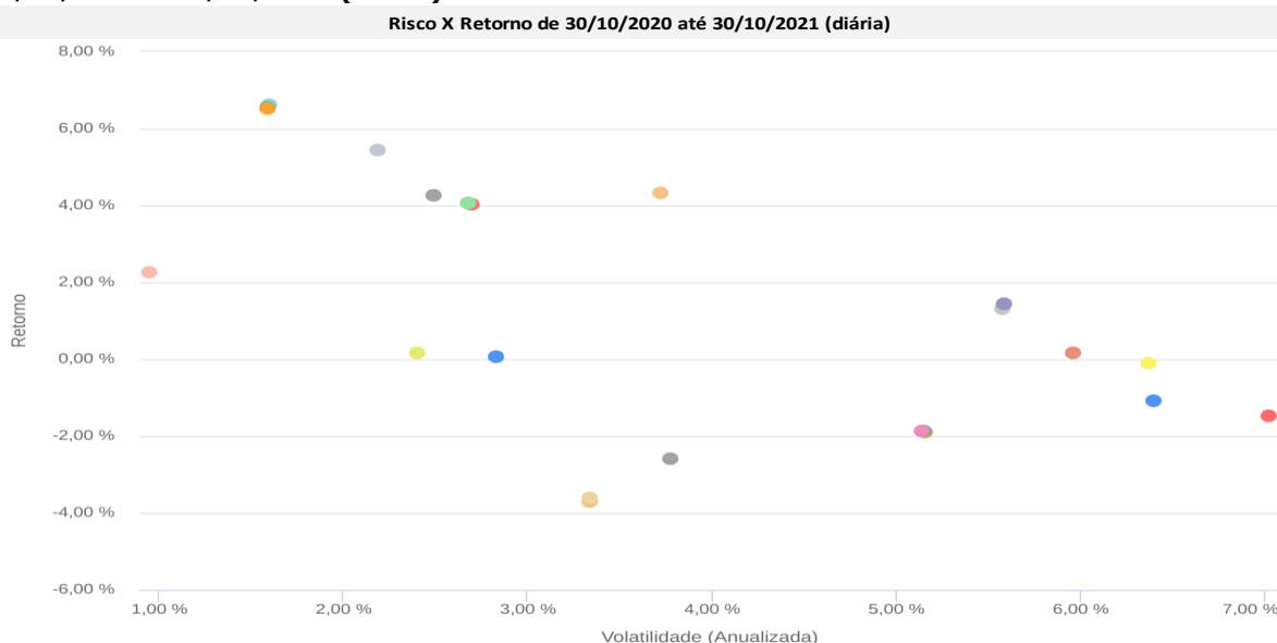
Gráfico 19: Risco x Retorno dos Fundos de Investimentos – Carteira FUNPREV: Renda Fixa 30/10/2020 a 30/10/2021 (diária).
